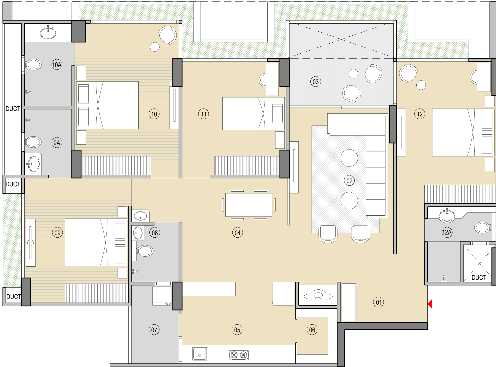
Type-B_L 4BHK_ Net area 144.88 sq.mt
