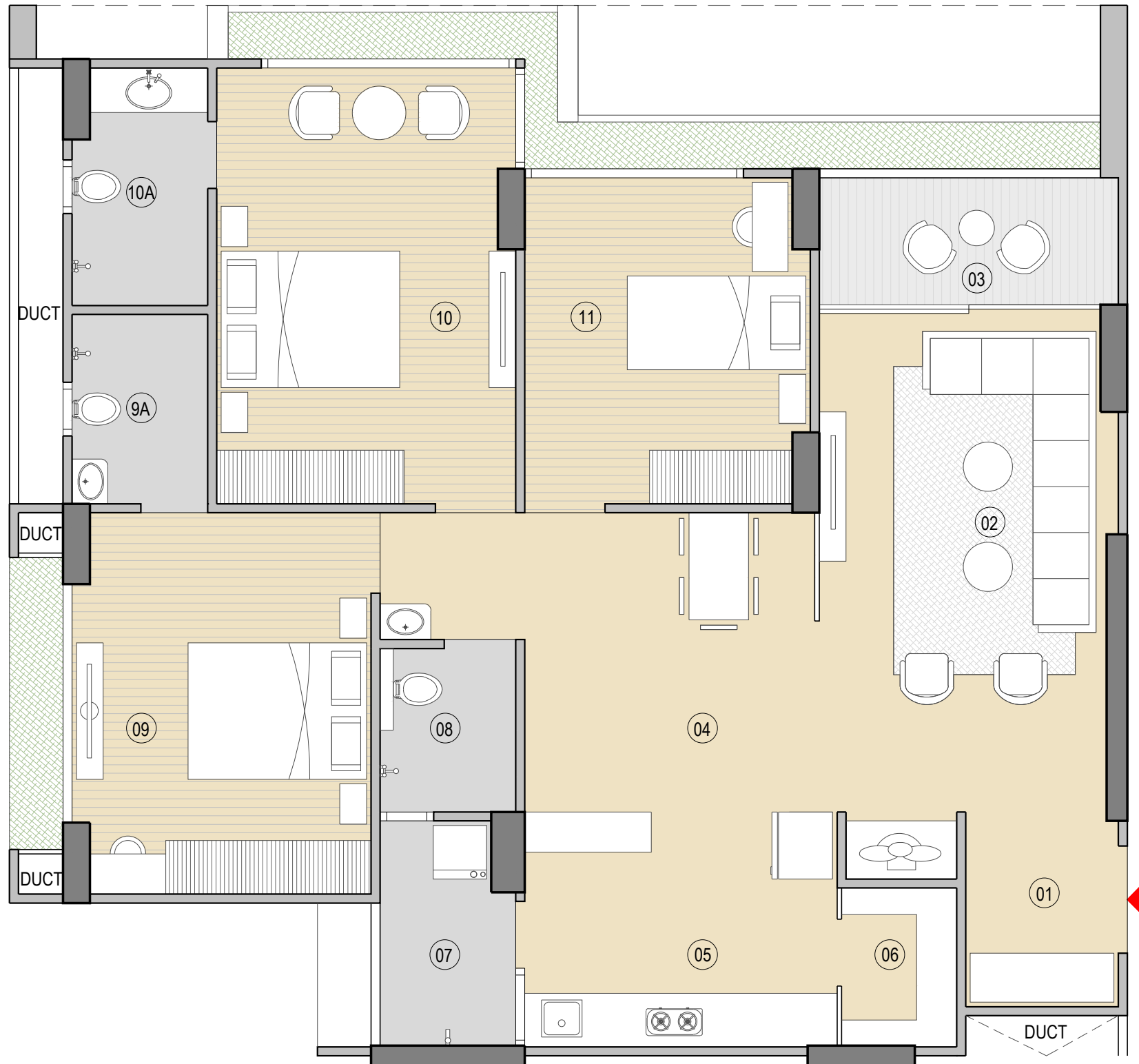
Type-C_N 3BHK_Net area 118.04 sq.mt
